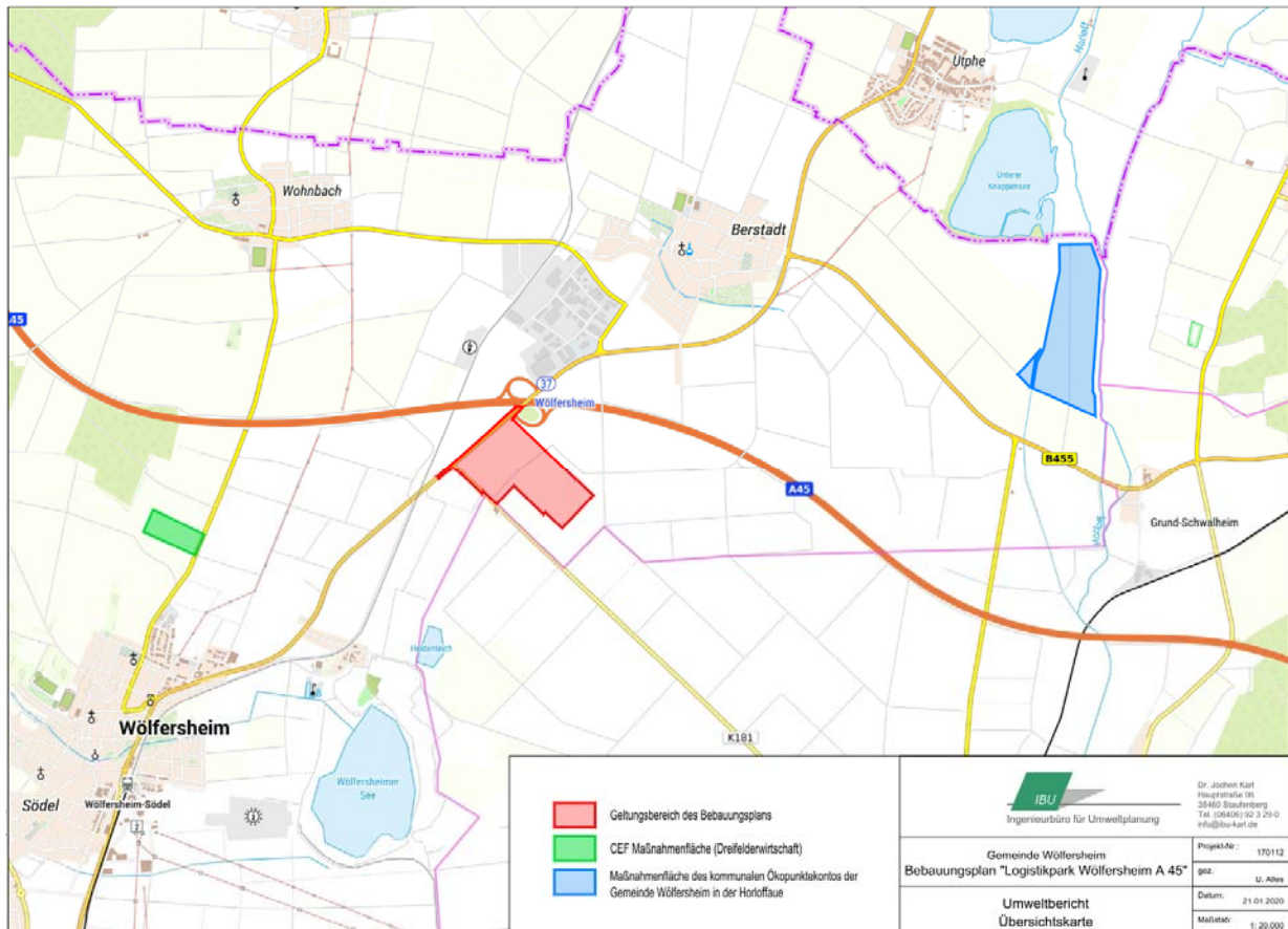
Abb. 9: Übersichtskarte Umweltbericht
